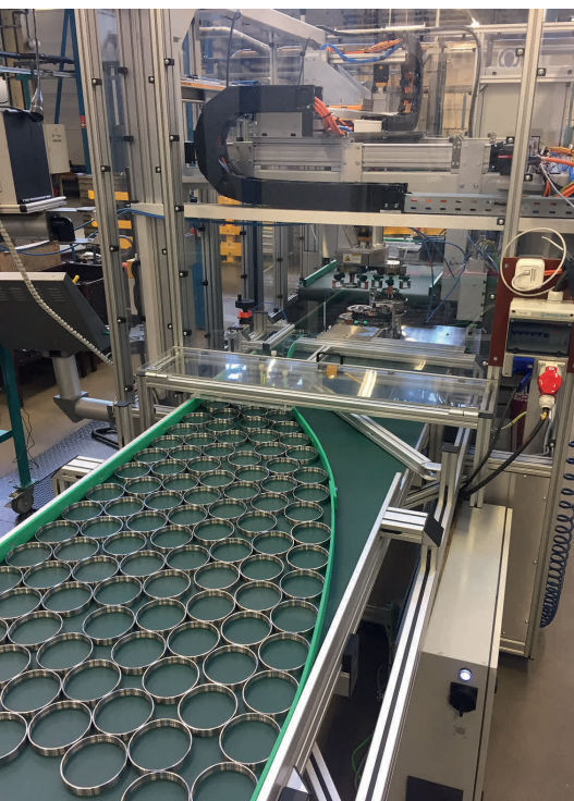
2 Prüfautomat QuaSor E zur Schleifbrandprüfung von Wälzlagerringen: Gesamtansicht mit Zuführband © imq
